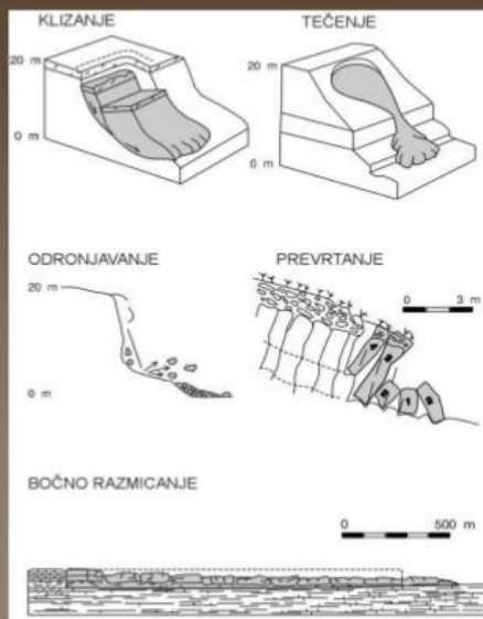
Slika: Tipovi klizišta
