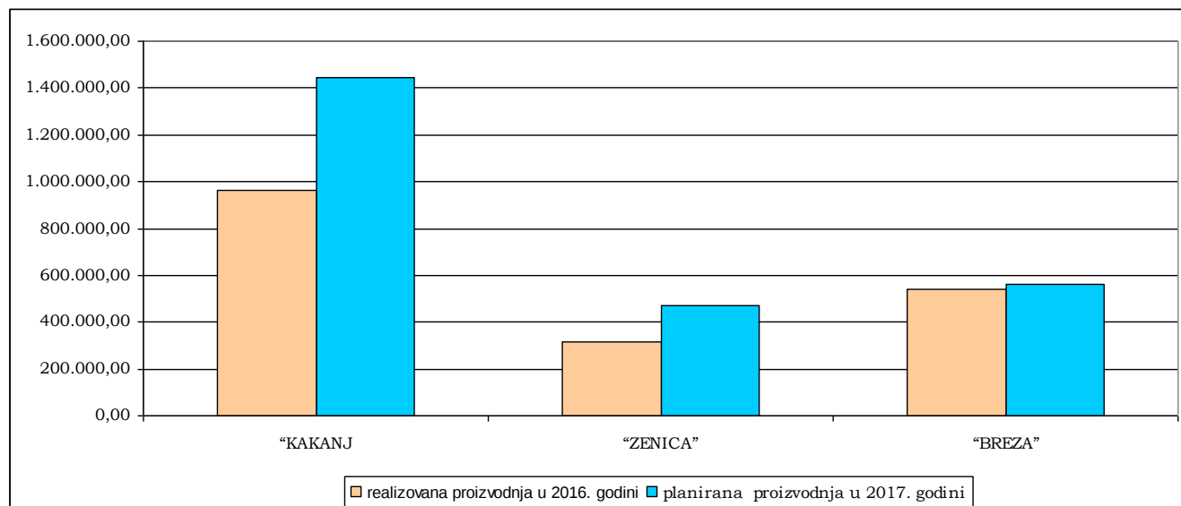
Dijagram 5. Proizvodnja uglja na području Zeničko-dobojskog kantona
