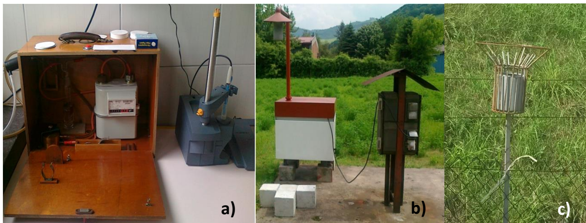
Slika 13. Uređaji za određivanje SO 2 (a), ULČ (b) i UTM (c) u zraku
