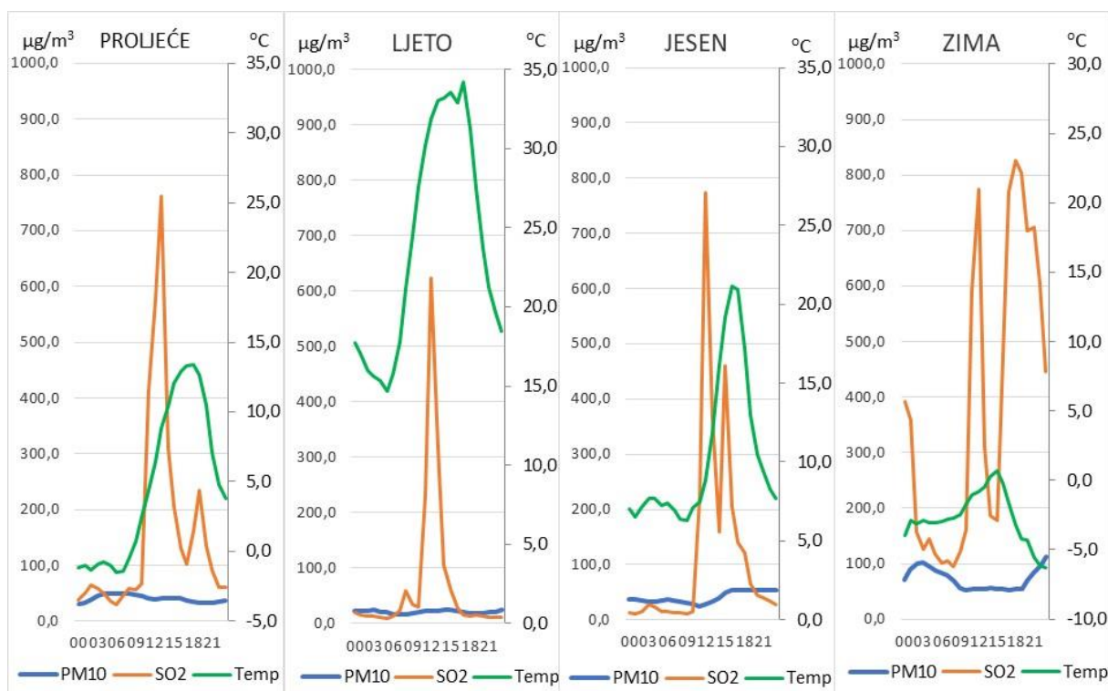
Slika 46. Dnevna dinamika koncentracija \text{SO}_2 i \text{PM}_{10} u odnosu na temperaturu zraka u Kaknju
