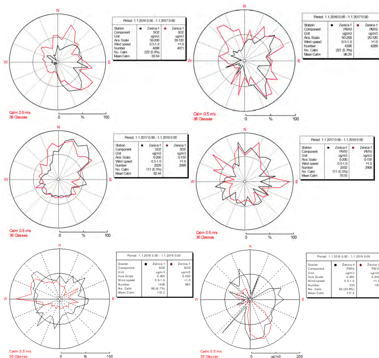
Slika 58. Ovisnost nivoa koncentracija \text{SO}_2 i \text{PM}_{10} o smjeru vjetra sa mjerne stanice Zenica-Centar
