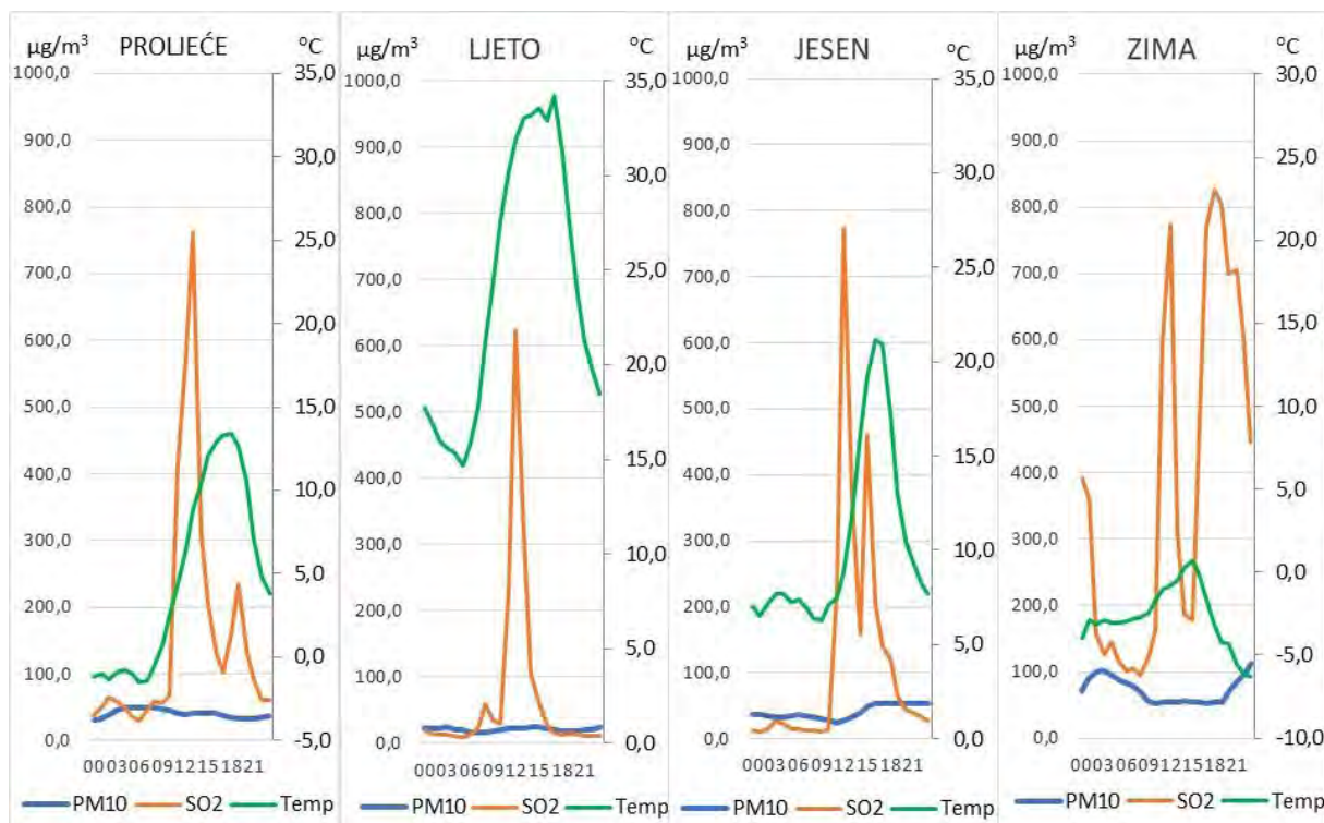
Slika 47. Dnevna dinamika koncentracija \text{SO}_2 i \text{PM}_{10} u odnosu na temperaturu zraka u Kaknju
