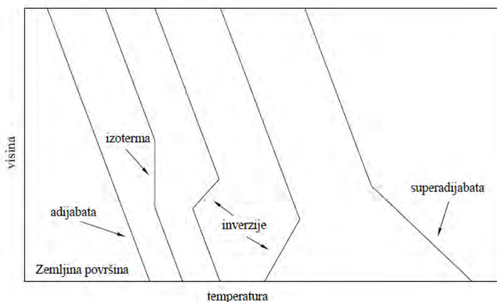
Slika 50. Karakteristične raspodjele temperature atmosfere u zavisnosti od visine
