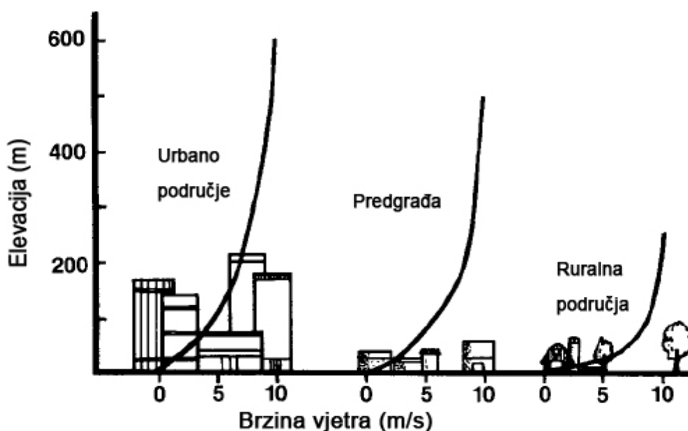
Slika 49. Vertikalni profili brzine vjetra s obzirom na tipove hrapavosti površine
