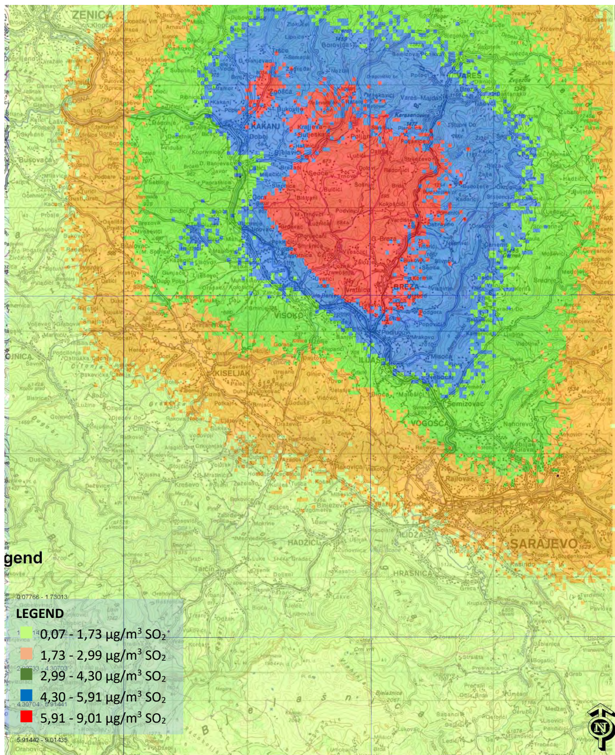
Slika 35. Disperzija \text{SO}_2 emitovana iz visokog dimnjaka TE Kakanj
